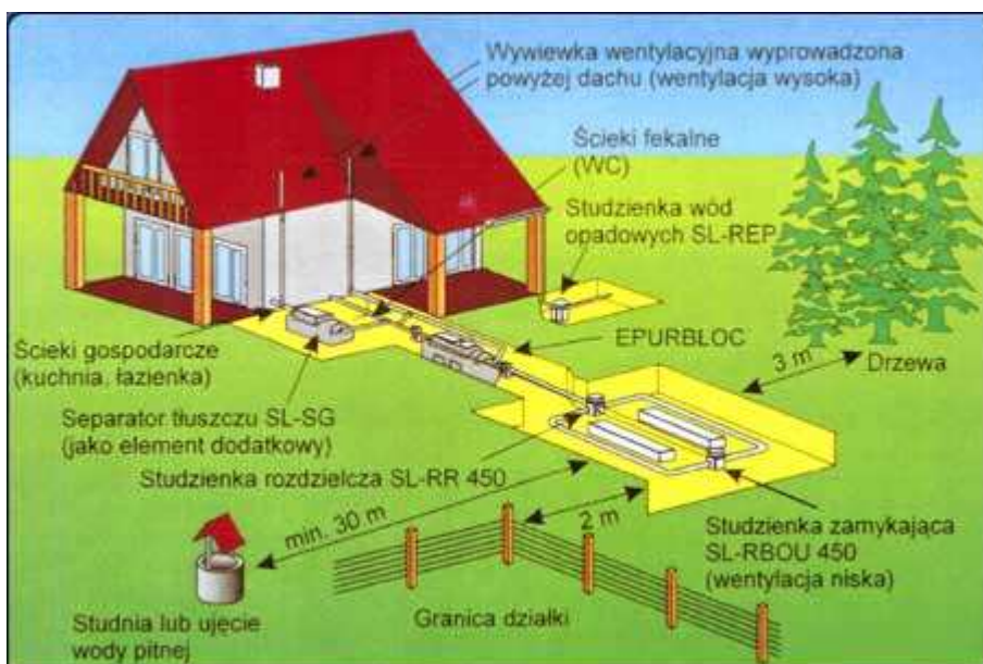
Schemat oczyszczania ścieków.
